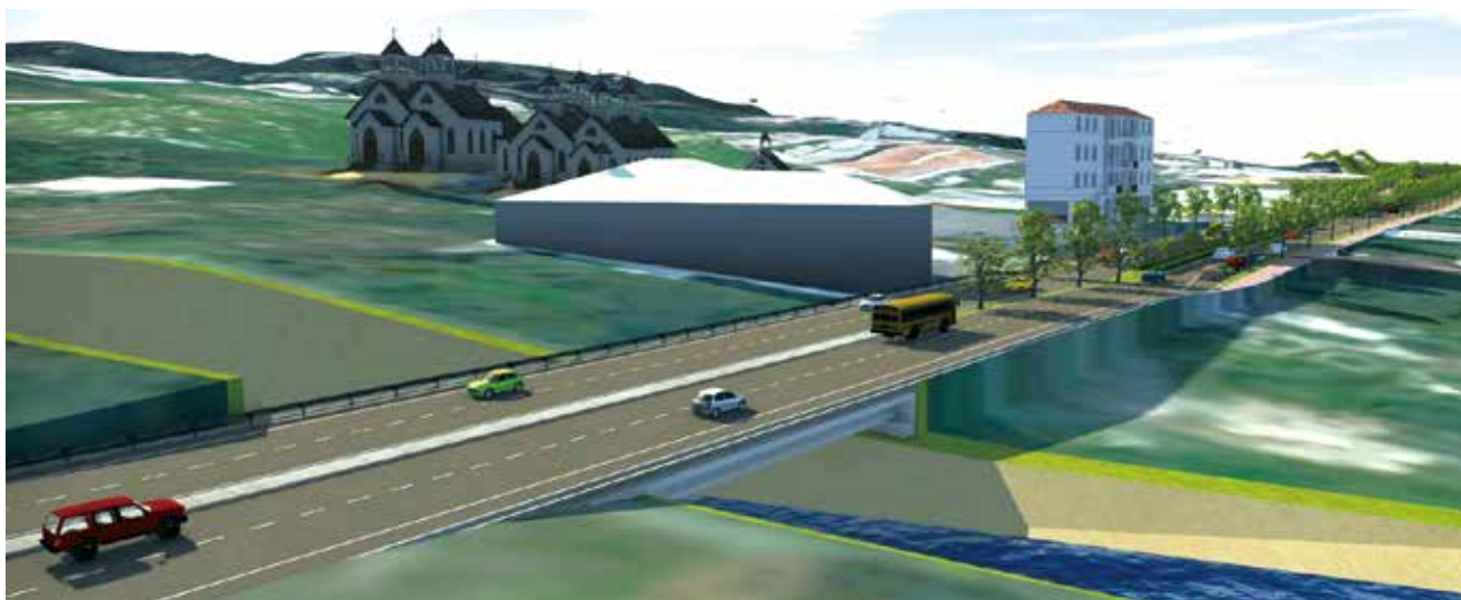
南投市 139 丙線 0K+000~1K+740 道路新建工程竣工模擬示意圖
