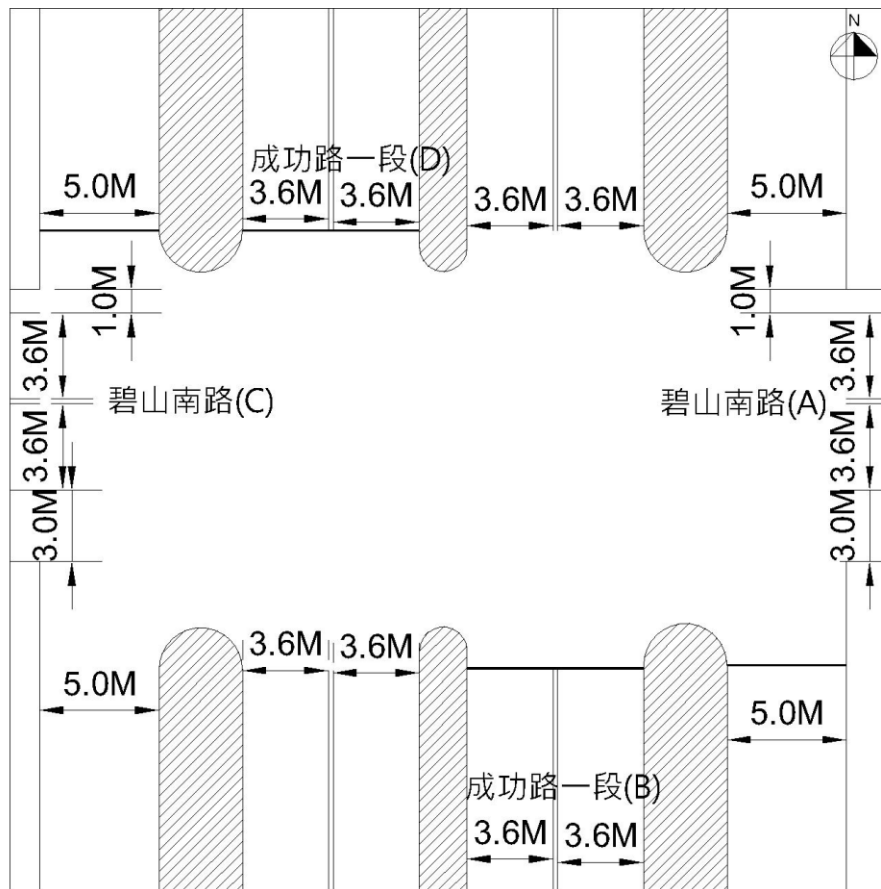
碧山南路/成功路一段路口簡圖
