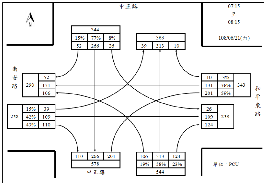
53. 南安路/中正路週五上午尖峰路口轉向圖
