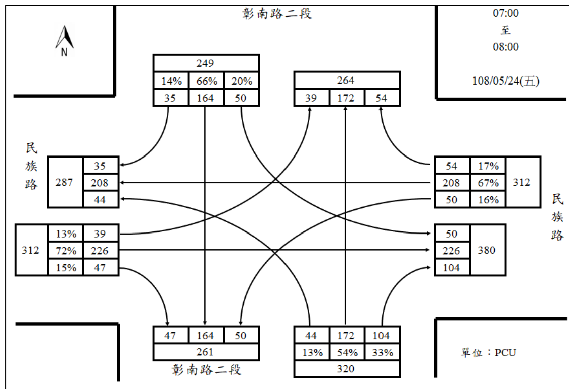
51.民族路/彰南路二段週五上午尖峰路口轉向圖
