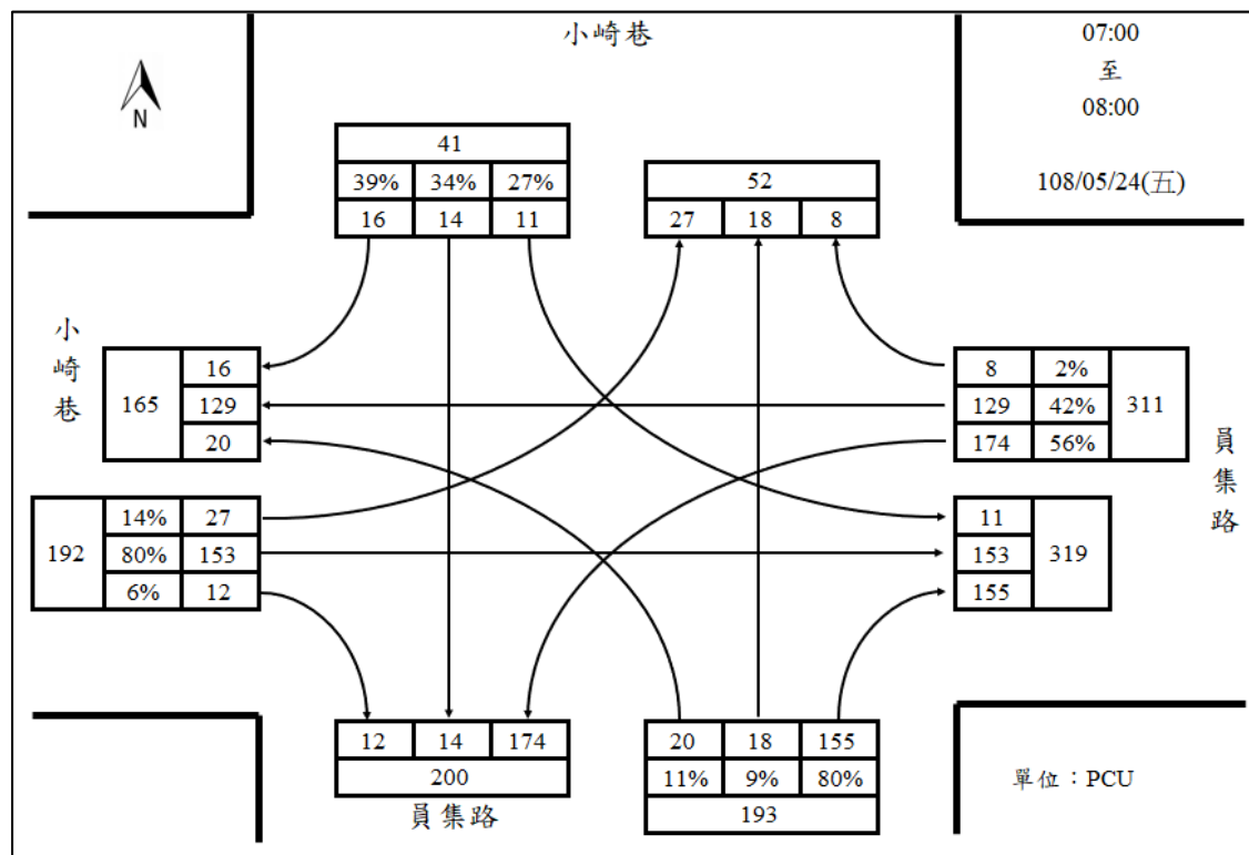
26.員集路/小崎巷週五上午尖峰路口轉向圖
