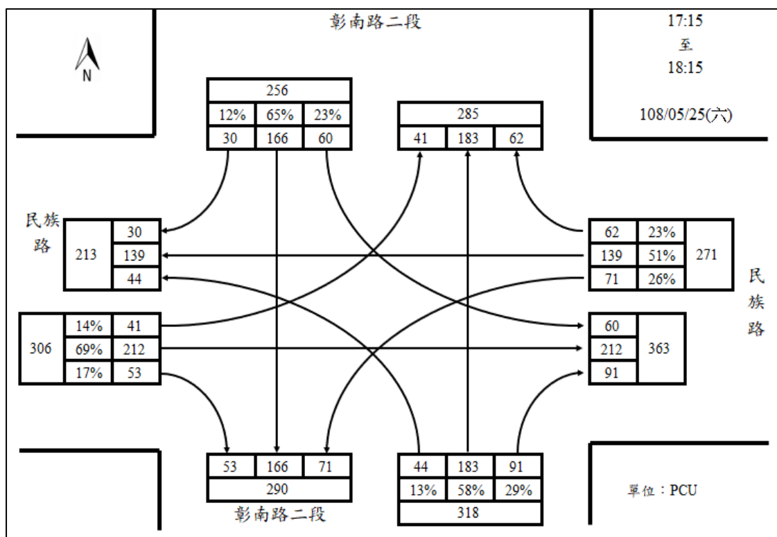
51.民族路/彰南路二段週六下午尖峰路口轉向圖
