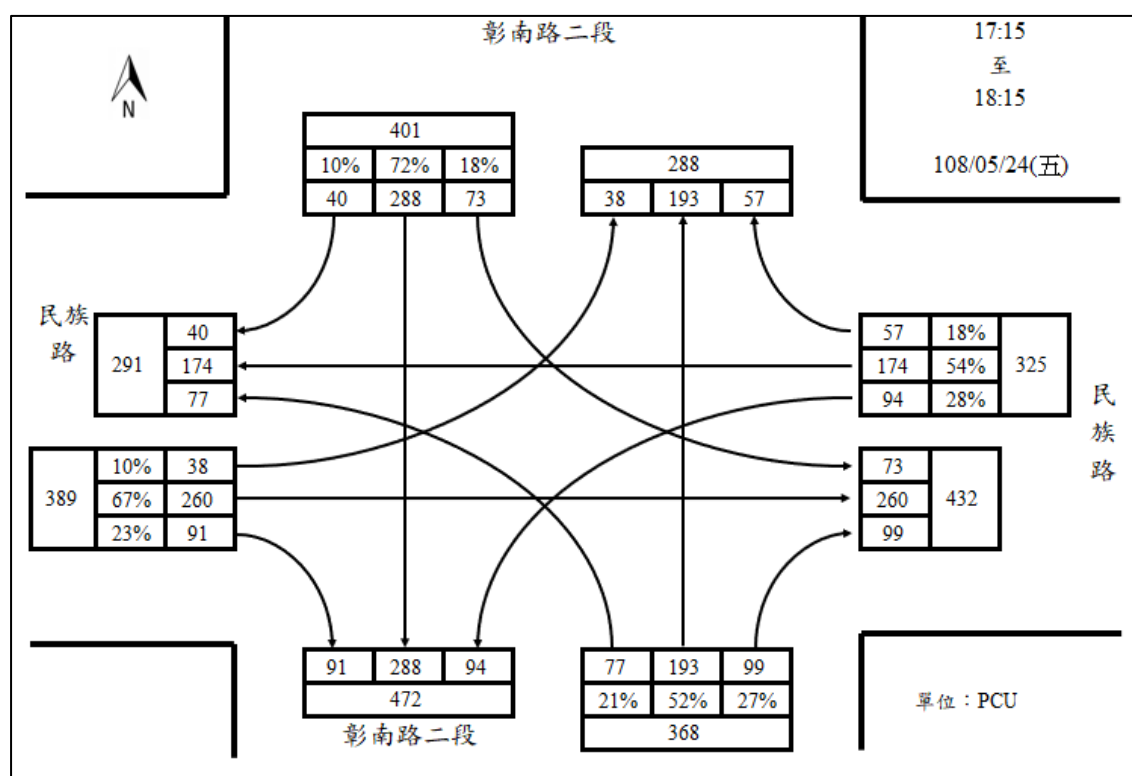
51.民族路/彰南路二段週五下午尖峰路口轉向圖
