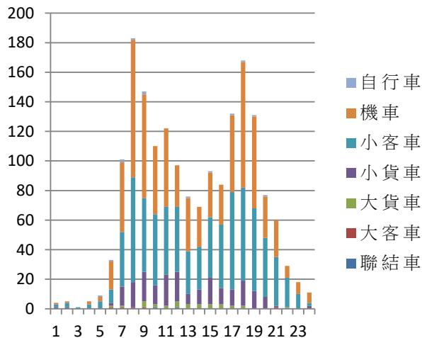
交通量組成長條圖
