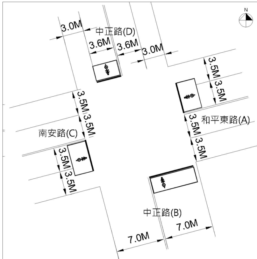
南安路/中正路路口簡圖
