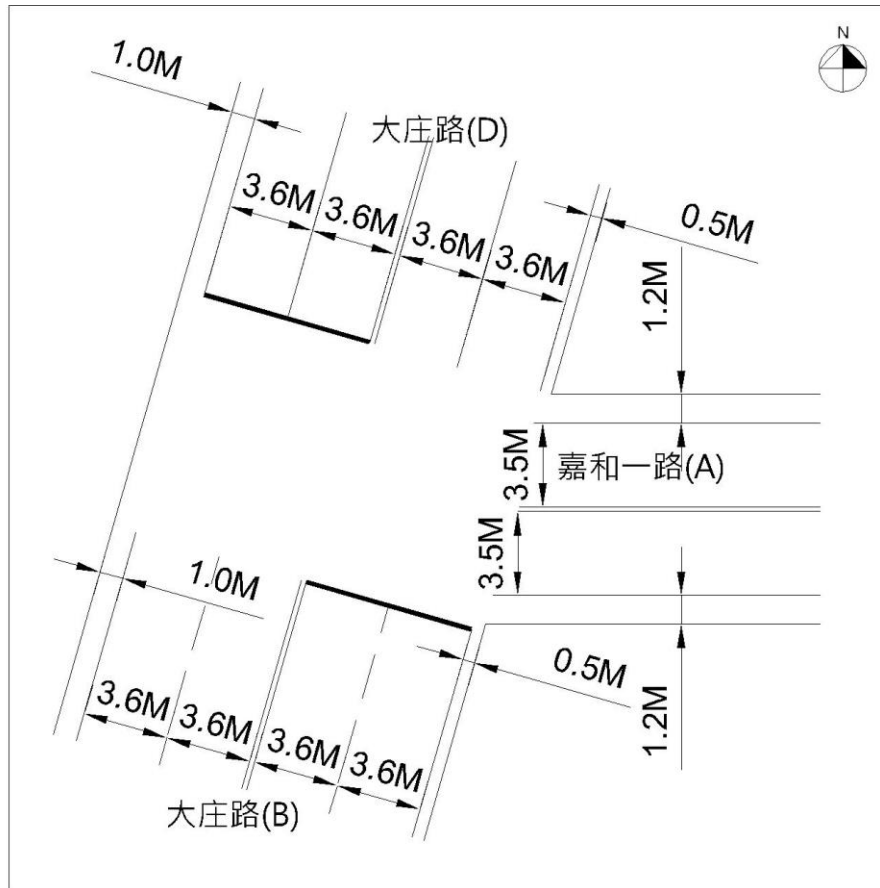
嘉和一路/大庄路路口簡圖
