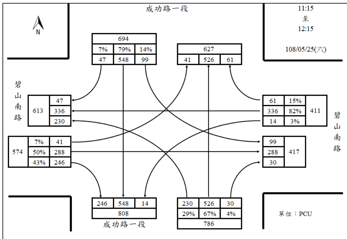
52. 碧山南路/成功路一段週六上午尖峰路口轉向圖
