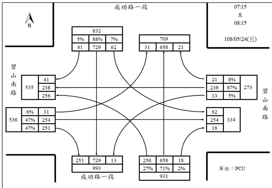
52. 碧山南路/成功路一段週五上午尖峰路口轉向圖
