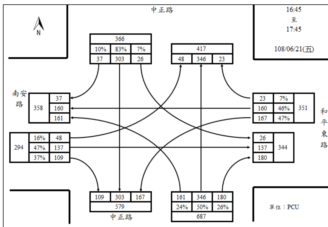
53. 南安路/中正路週五下午尖峰路口轉向圖
