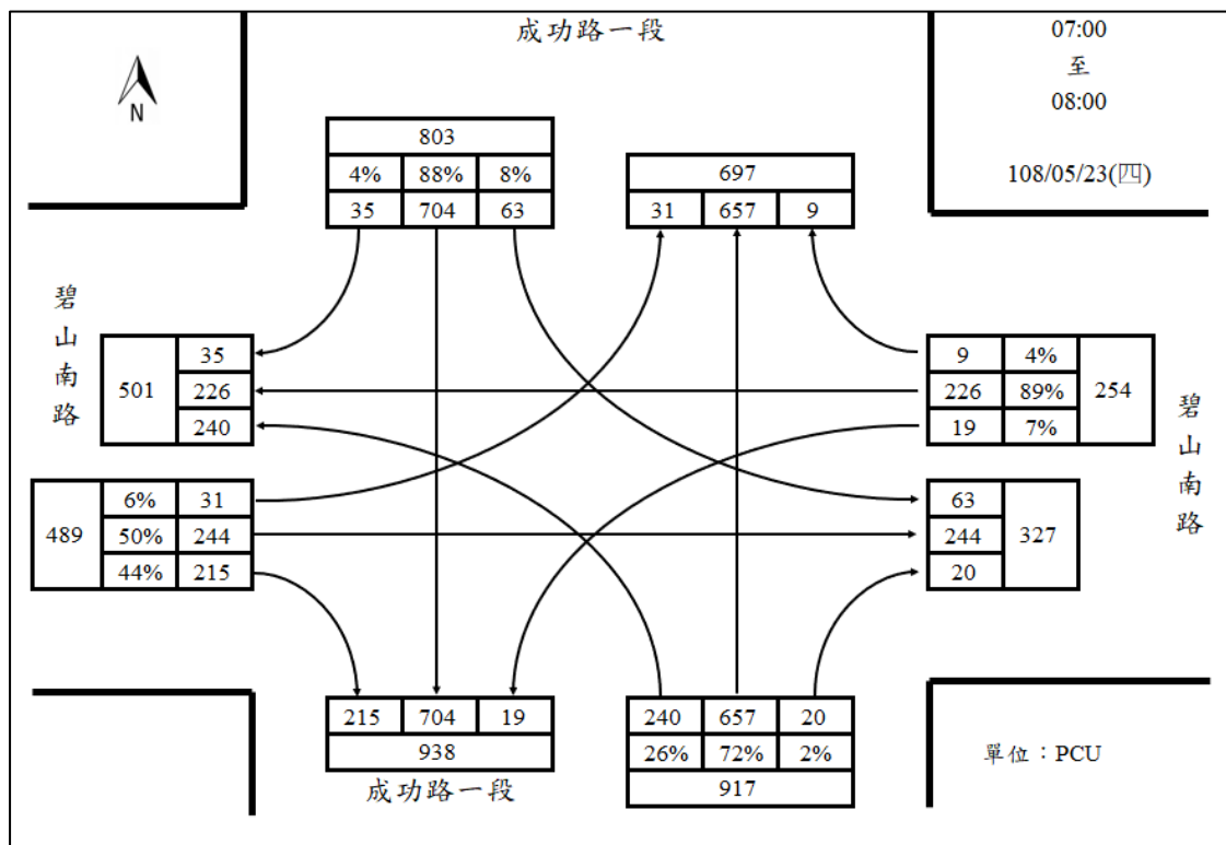
52.碧山南路/成功路一段週四上午尖峰路口轉向圖
