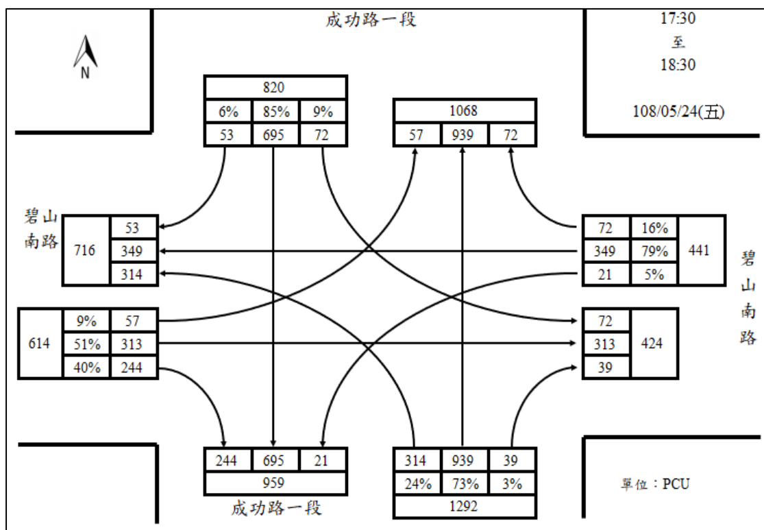
52. 碧山南路/成功路一段週五下午尖峰路口轉向圖
