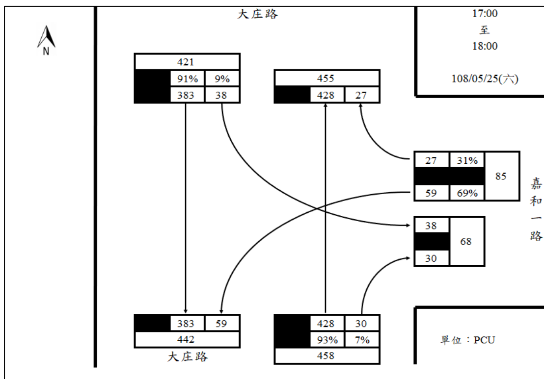
23.嘉和一路/大庄路週六下午尖峰路口轉向圖
