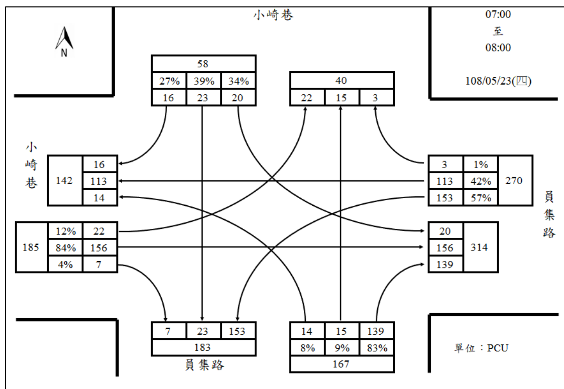
26.員集路/小崎巷週四上午尖峰路口轉向圖
