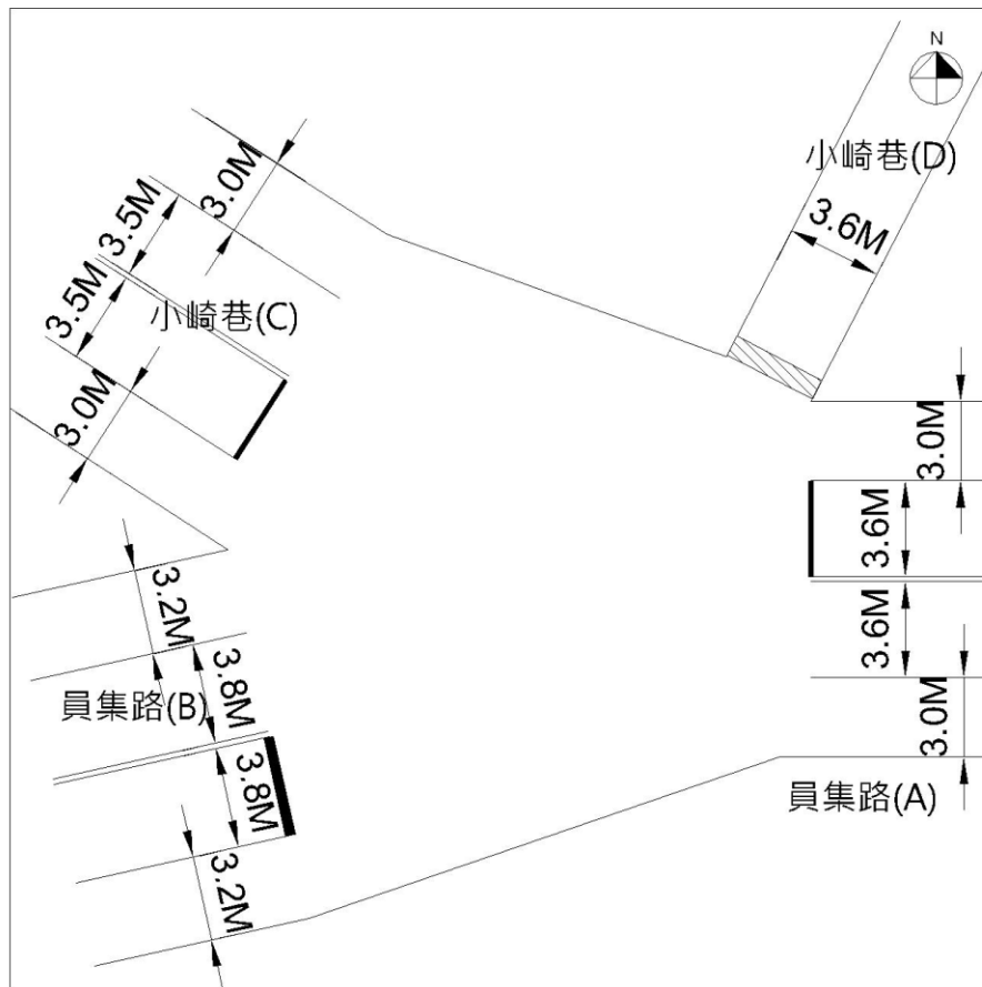
員集路/小崎巷口簡圖
