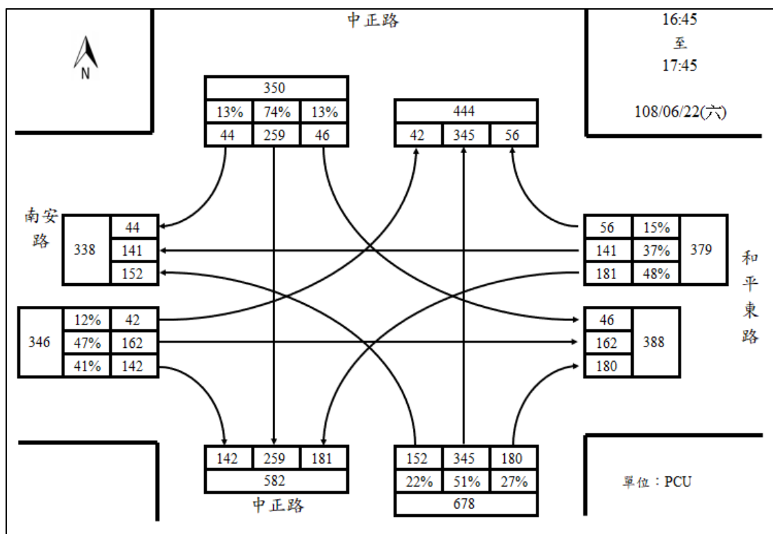
53. 南安路/中正路週六下午尖峰路口轉向圖
