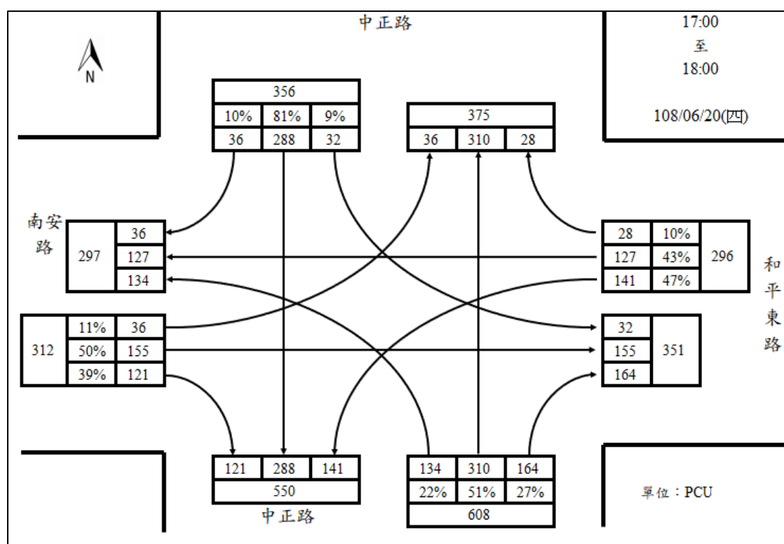
53.南安路/中正路週四下午尖峰路口轉向圖
