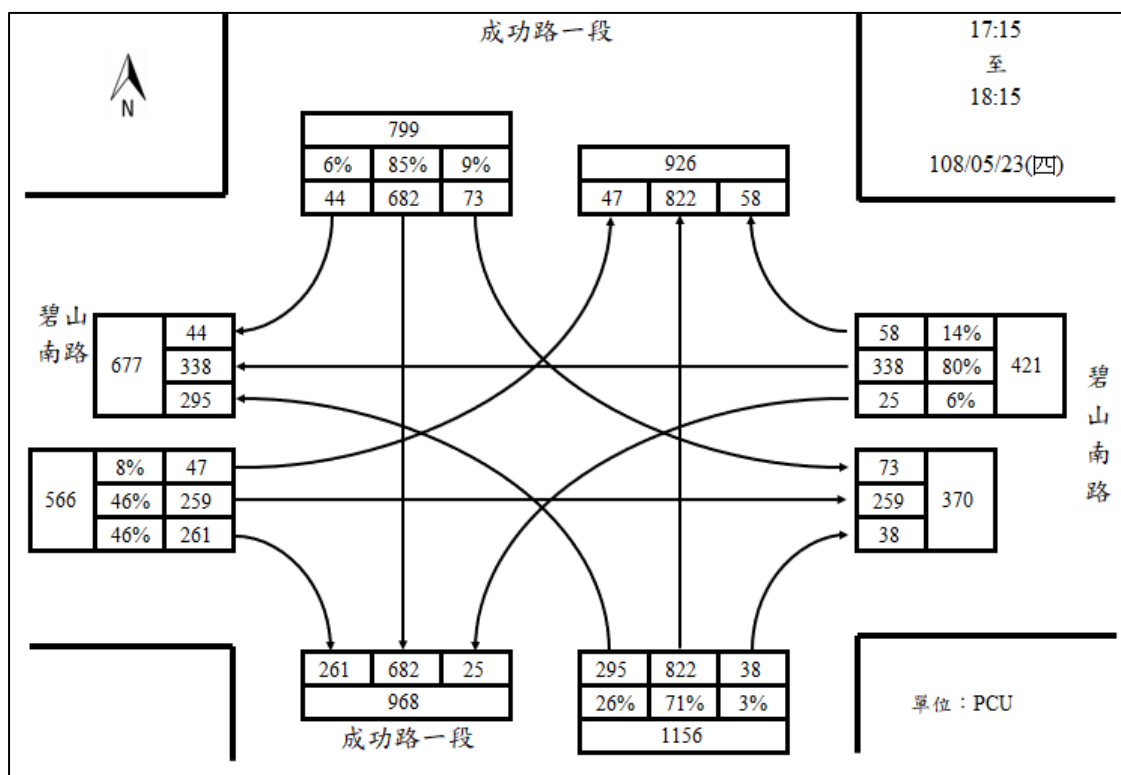
52.碧山南路/成功路一段週四下午尖峰路口轉向圖
