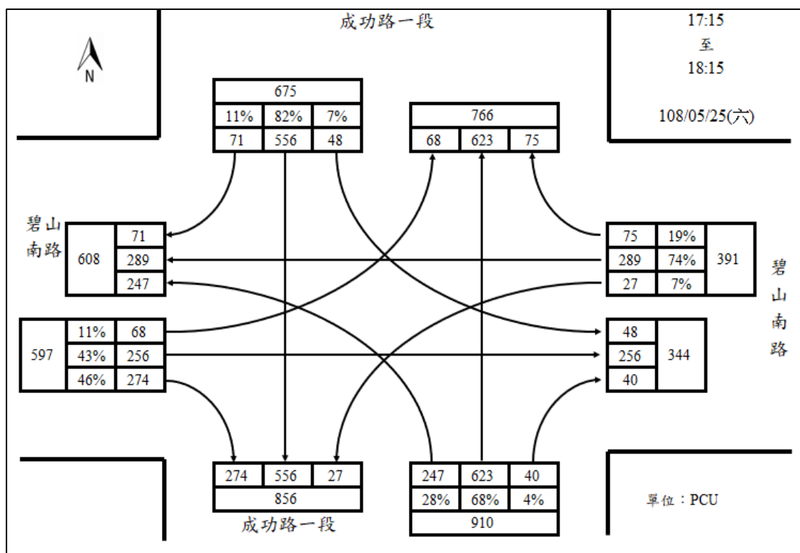
52. 碧山南路/成功路一段週六下午尖峰路口轉向圖
