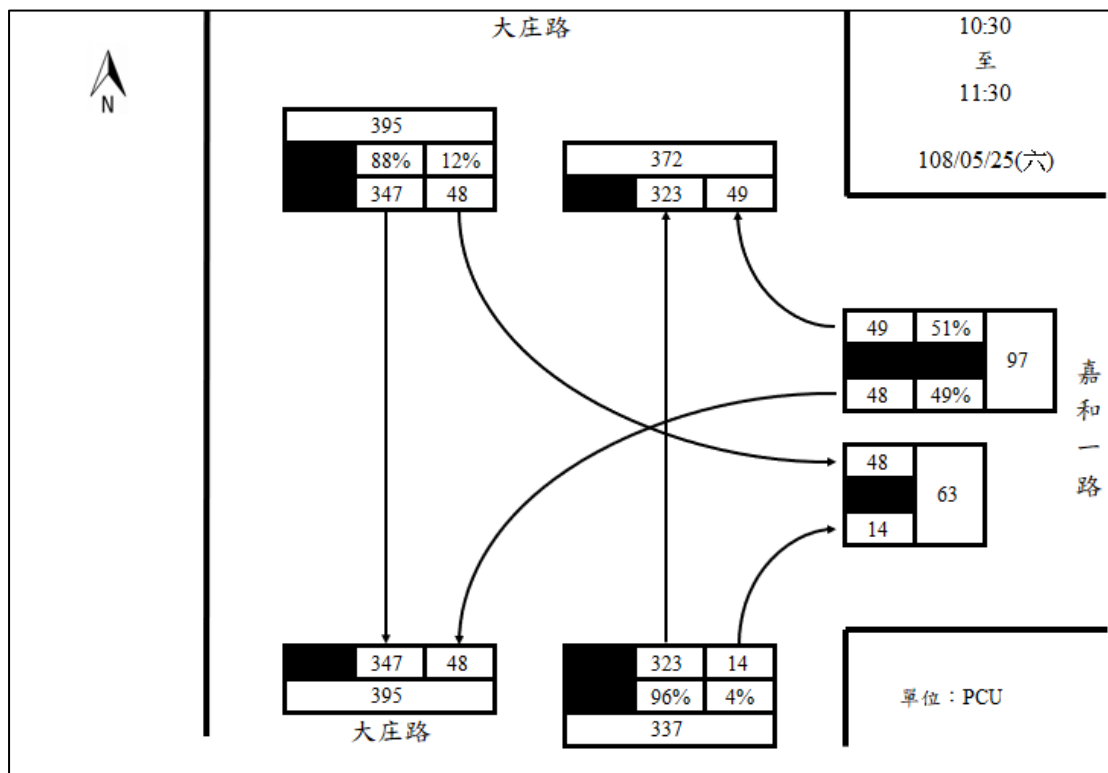
23.嘉和一路/大庄路週六上午尖峰路口轉向圖
