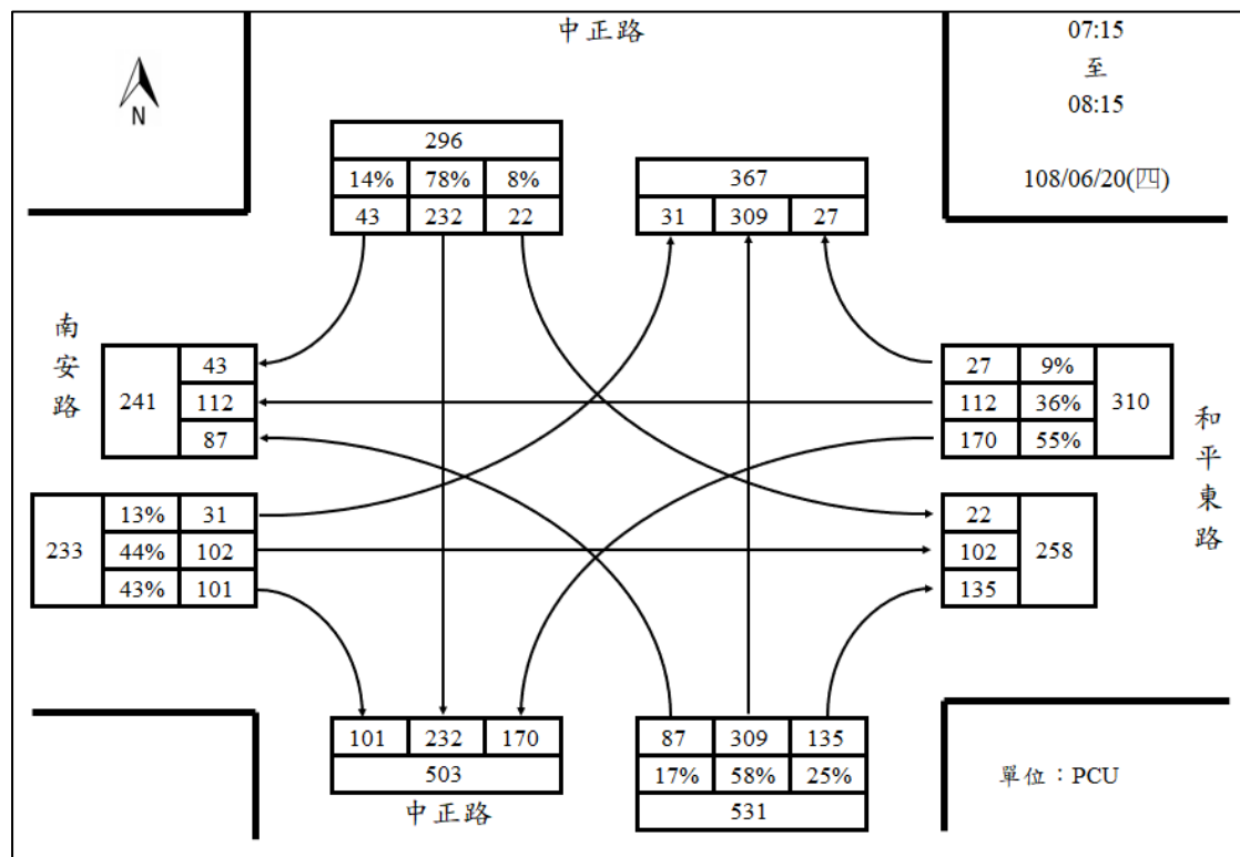
53.南安路/中正路週四上午尖峰路口轉向圖
