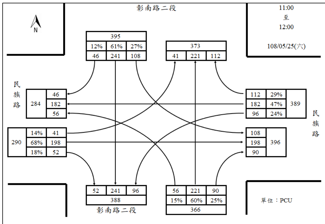
51.民族路/彰南路二段週六上午尖峰路口轉向圖
