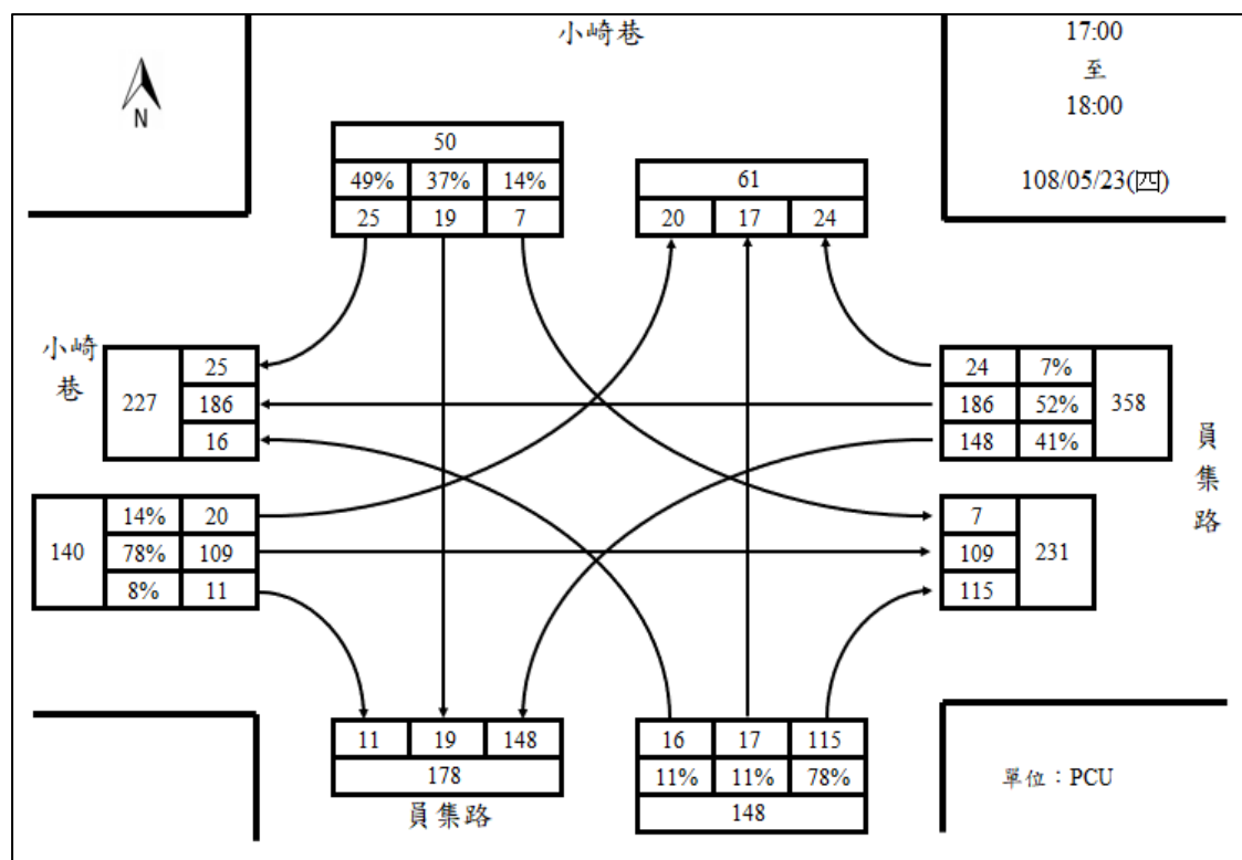
26.員集路/小崎巷週四下午尖峰路口轉向圖
