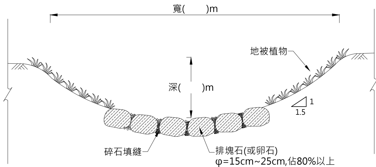
複式草溝示意圖
