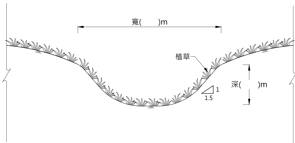
草溝示意圖
