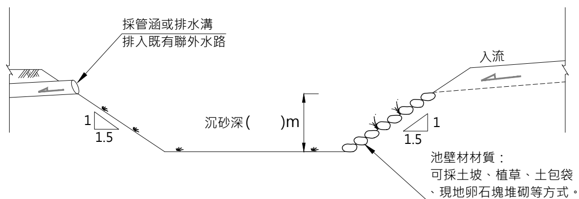
簡易農地沉砂池剖面示意圖
