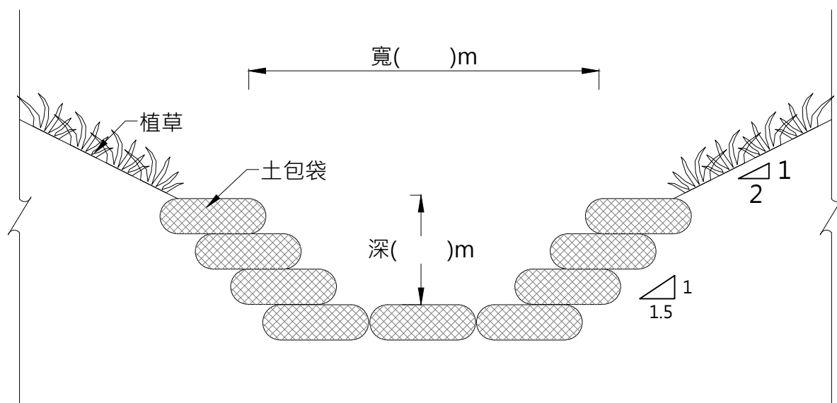
土包袋溝示意圖
