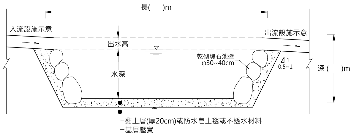
農塘剖面示意圖
