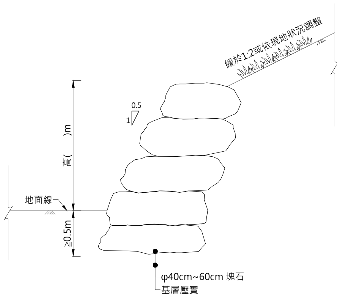
乾砌石擋土牆示意圖
