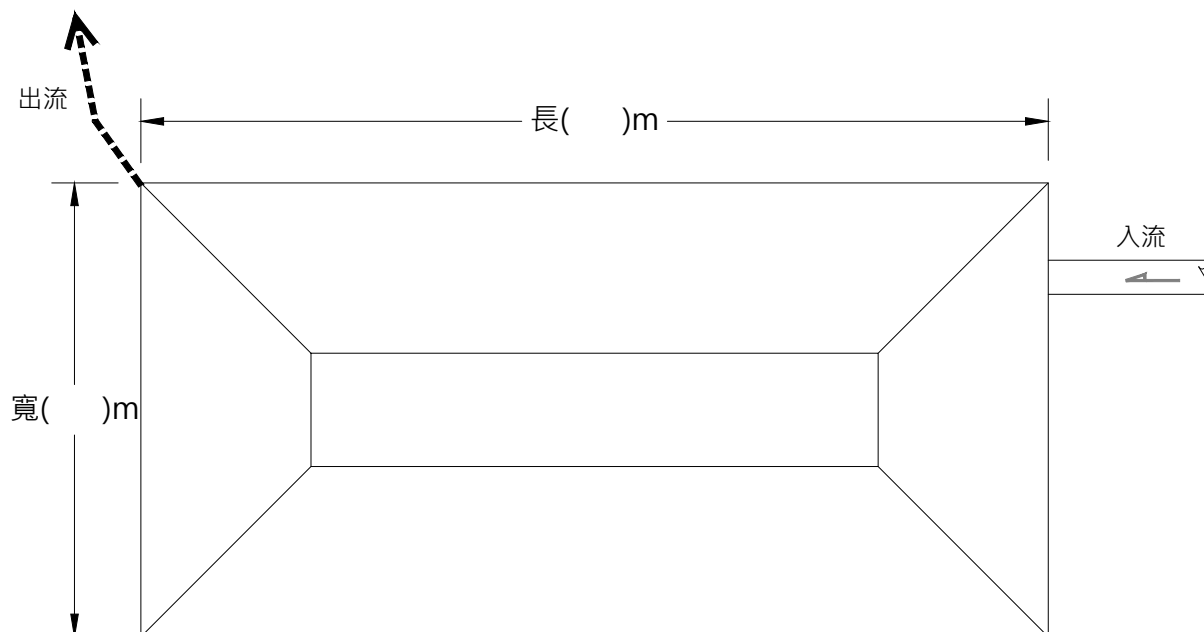
簡易農地沉砂池平面示意圖
