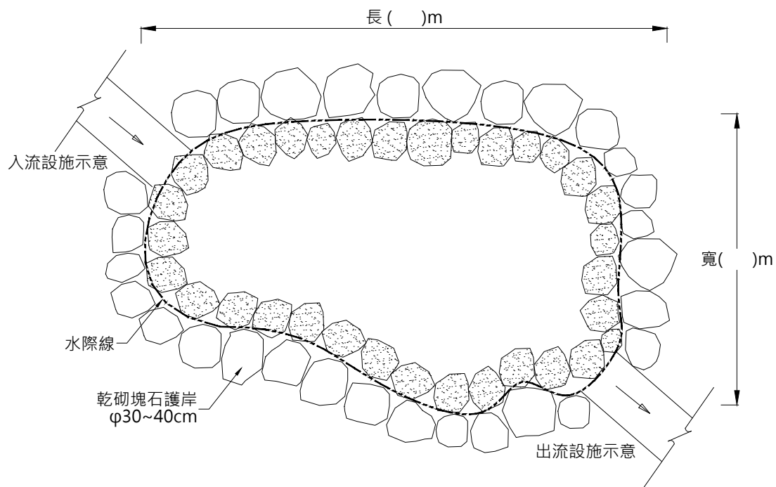
農塘平面示意圖
