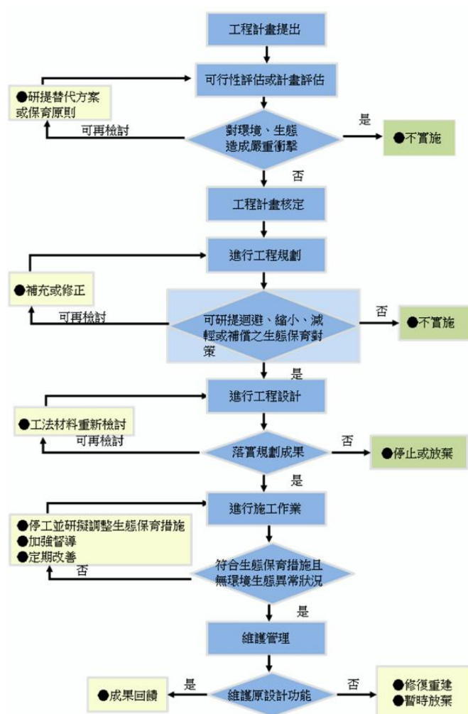
圖 3-1 公共工程生態檢核作業流程圖
