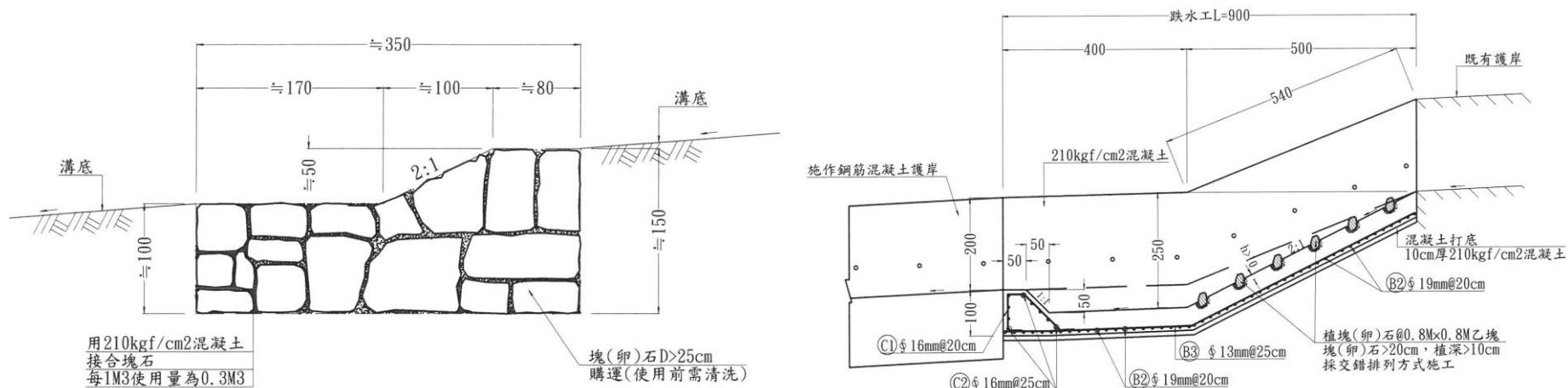
圖 4-11 北港溪排水幹線-2 固床工(左)與跌水工(右)設計圖
