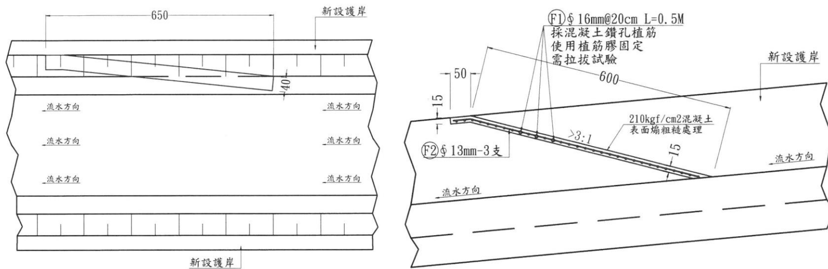
圖 4-12 北港溪排水幹線-2 動物坡道平面(左)與立面(右)圖
