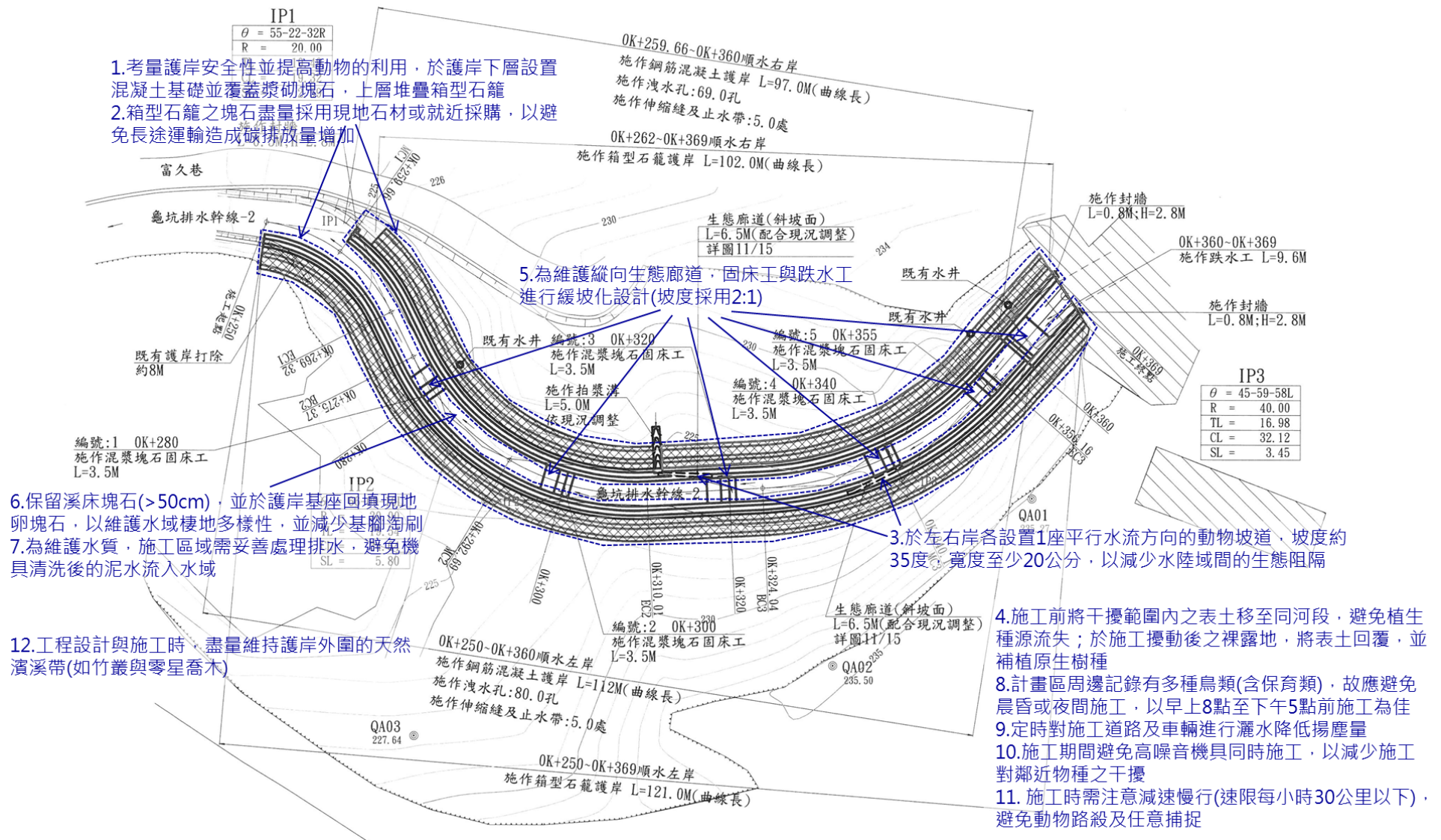
圖 4-11 龜坑排水幹線-2 生態保育措施平面圖
