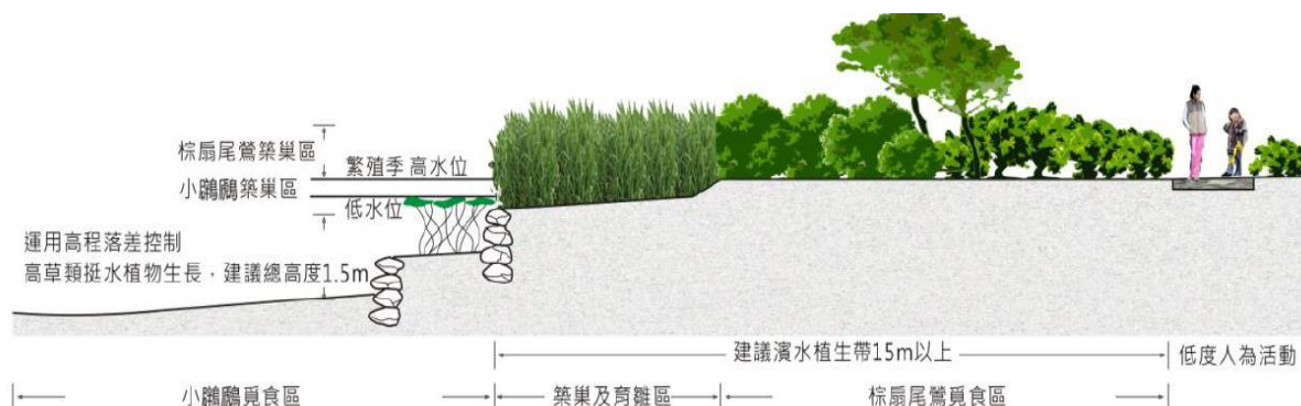
圖 3-6 濱水高草區繁殖類棲地設計參考示意圖
