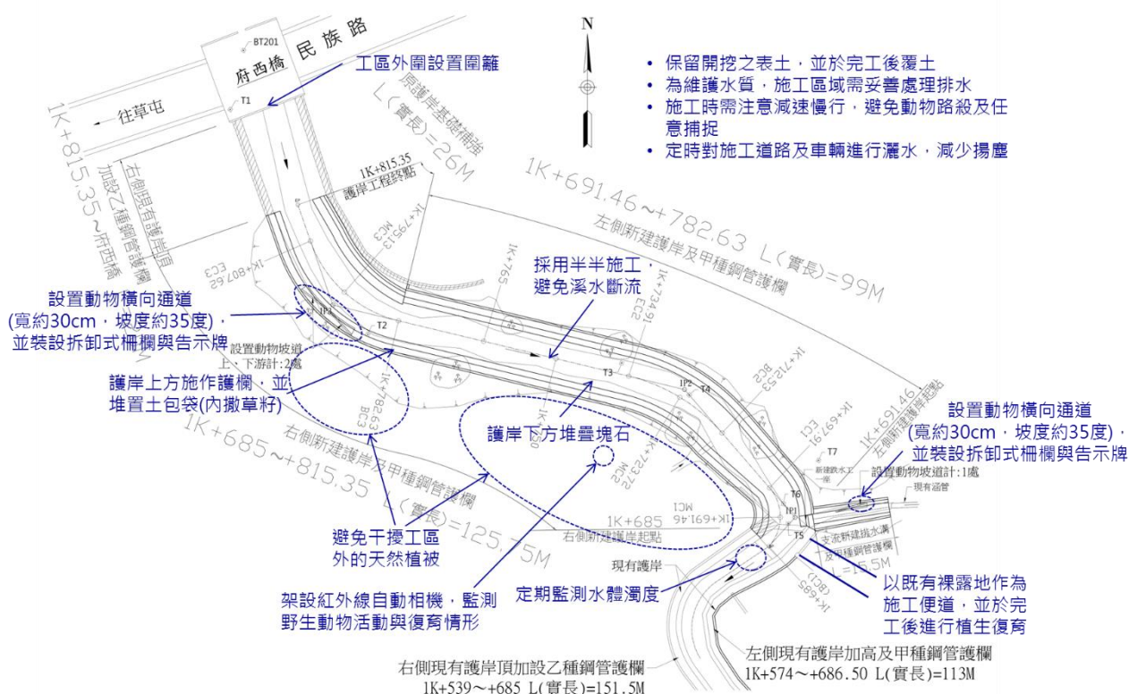
圖 3-7 111 頭前厝排水分線護岸應急工程(第二期)生態保育對策圖
